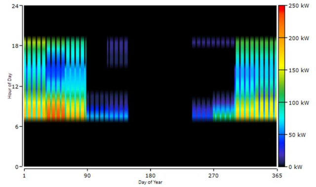
Fig. 2. Thermal demand.
