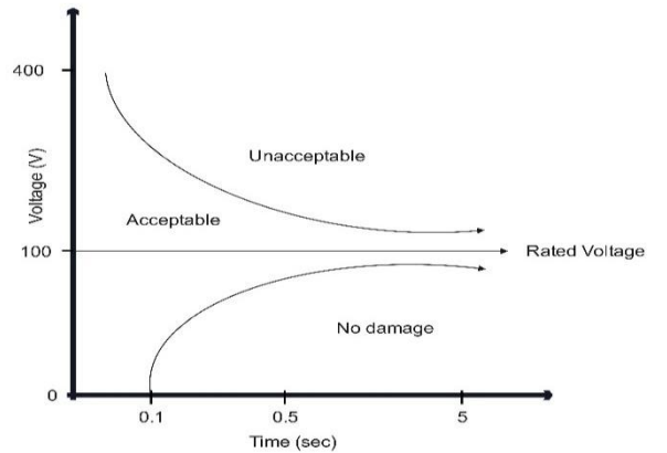
Fig.4 CBEMA curve.
